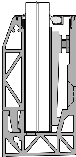
CACHE CÔTÉ VIDE CF-100
