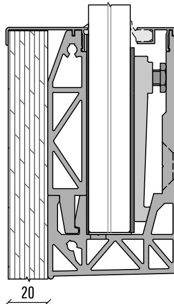
CACHE CÔTÉ VIDE CF-120
