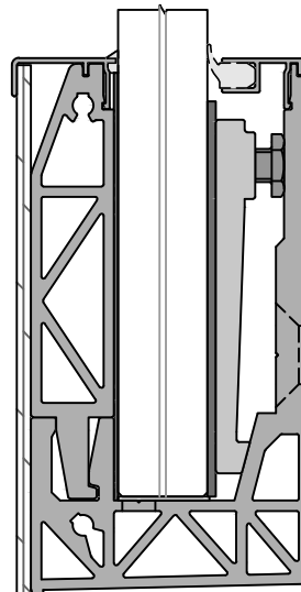
CACHE CÔTÉ VIDE CF-103
