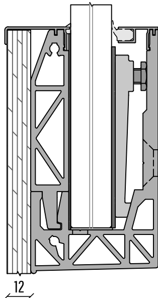
CACHE CÔTÉ VIDE CF-112
